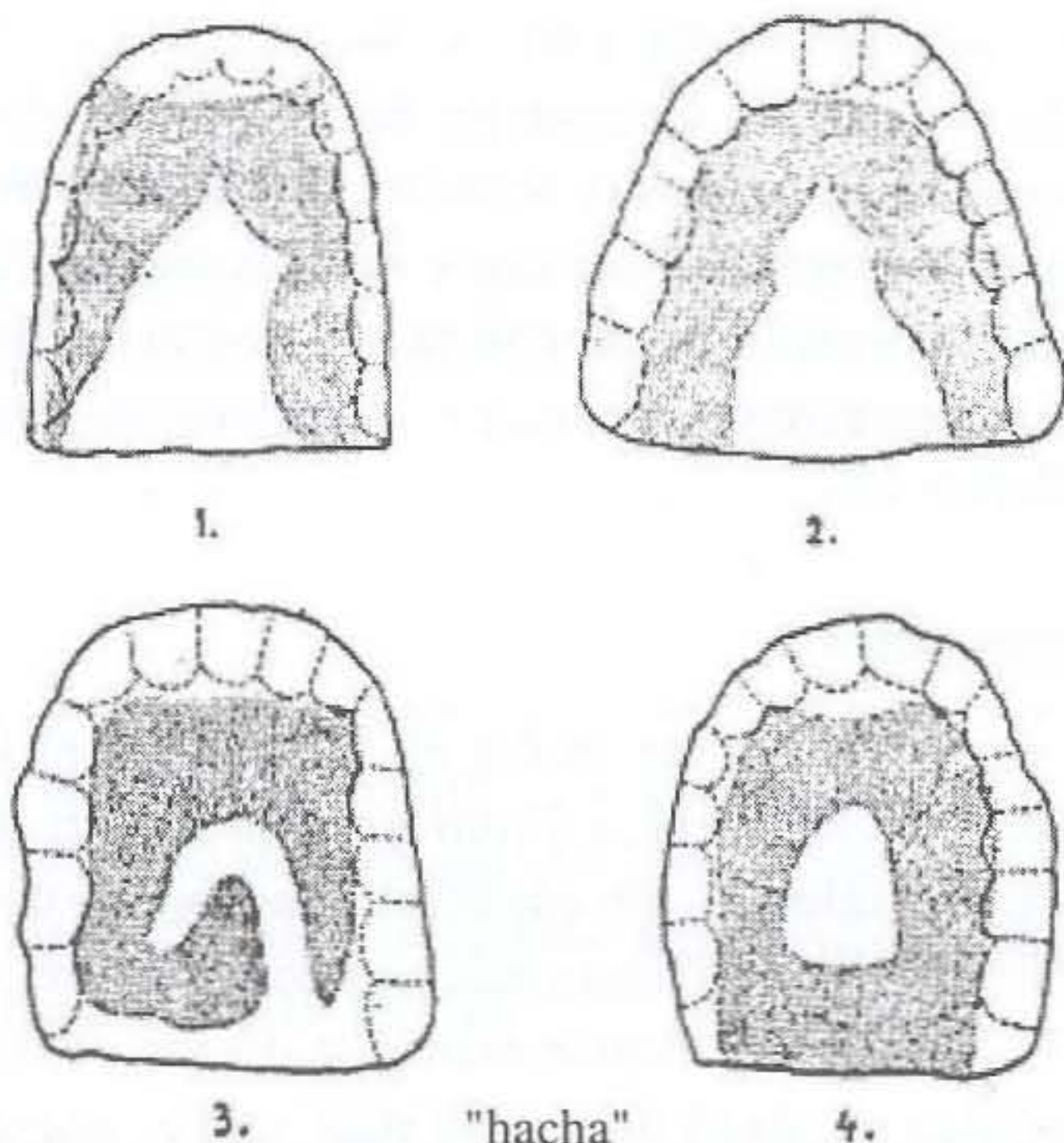
Variantes de ch : 1, africada, Lares; 2, africada, San Germán; 3, adherente, Bayamón; 4, adherente, Caguas.
