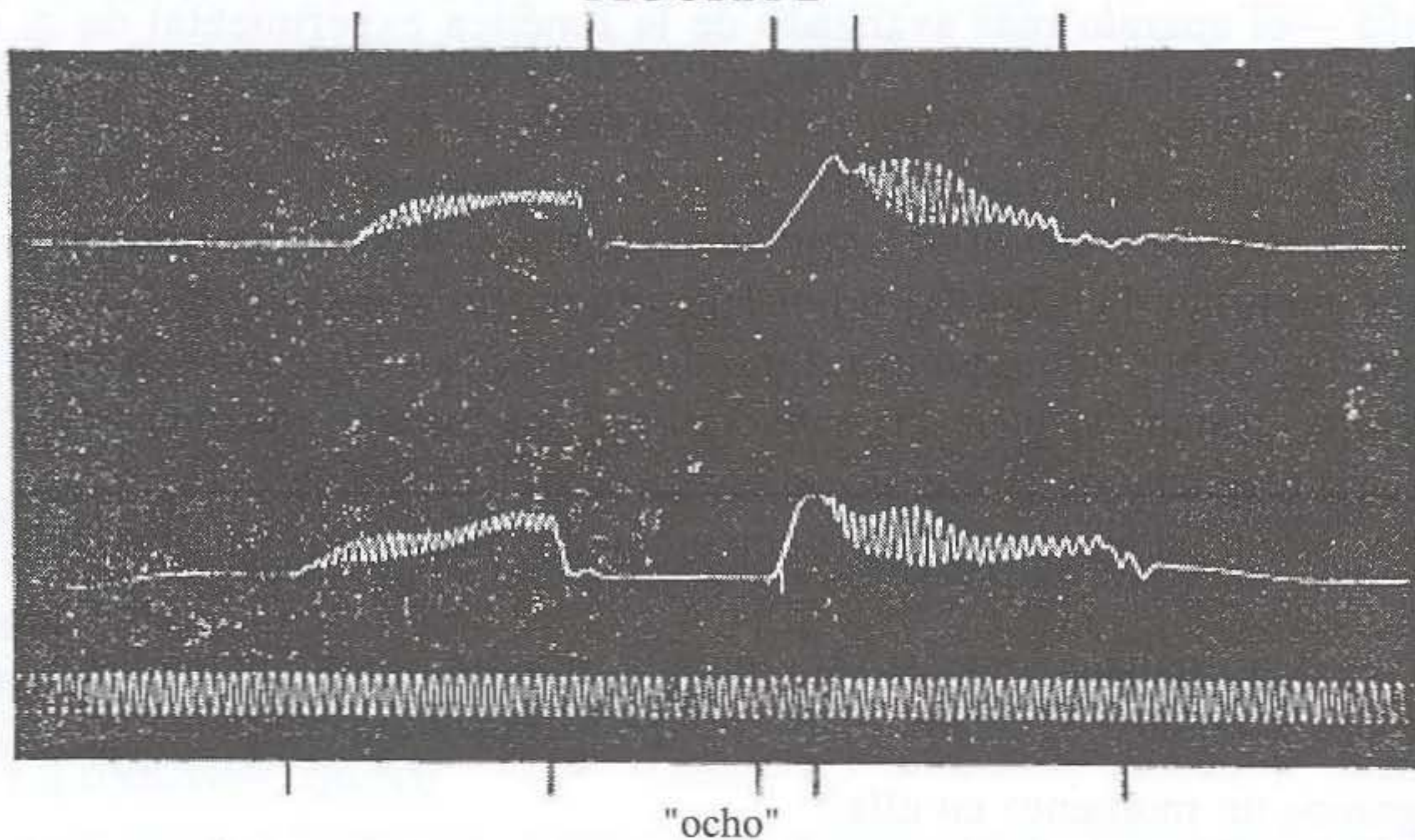
Duración total de la ch desde el primer punto de oclusión en ambas variantes, 21 c.s. En la primera, oclusión, 14; fricación, 7. En la segunda, oclusión, 17; fricación, 4. Diapasón: 200 v.d.
